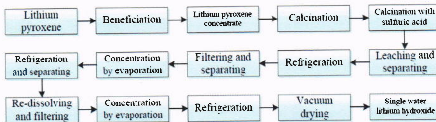
Cuadro 11 Método de Ácido Sulfúrico desde Concentrado de Mineral
