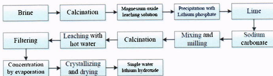
Cuadro 12 Método de Cal desde Concentrado de Salmuera
