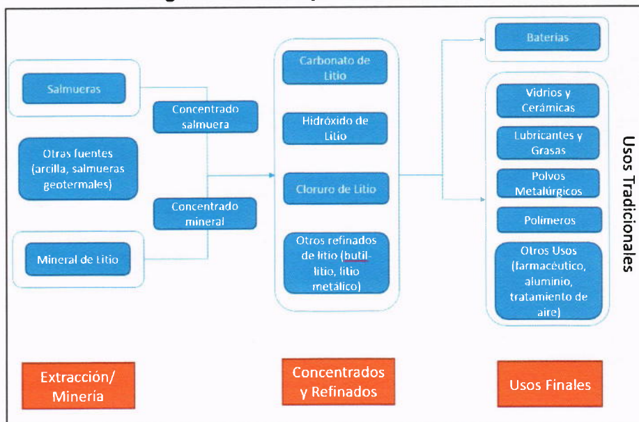
Cuadro 2 Diagrama de las etapas de la industria del litio
